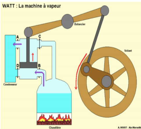
WATT : La machine à vapeur
